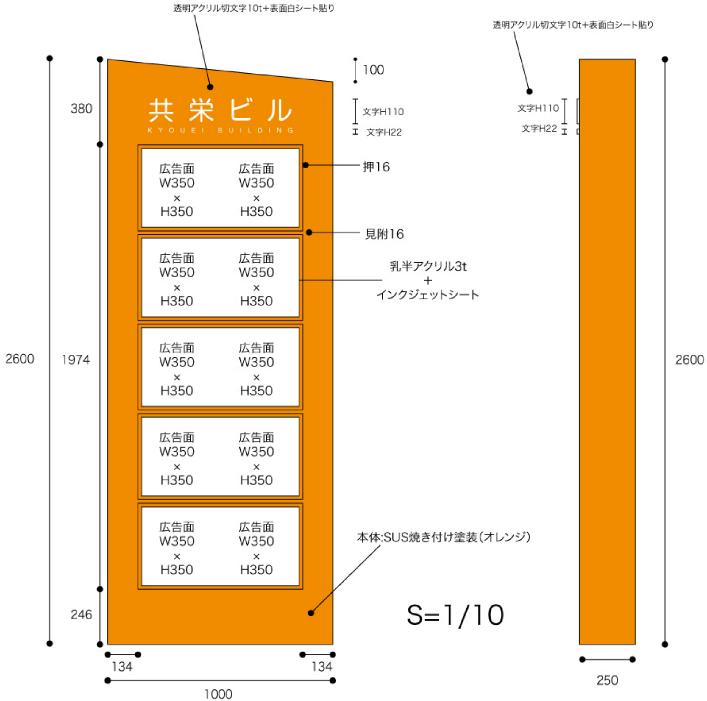
正面図
